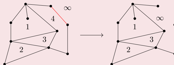
مثالی از روند استقرایی استفاده شده در اثبات
